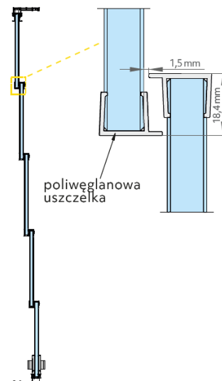
RZUT Z GÓRY SYSTEM Z USZCZELKĄ MIĘDZYSZYBOWĄ
