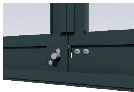
Zamek dolny samozatraskowy
