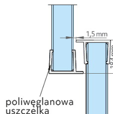
RZUT Z GÓRY SYSTEM Z USZCZELKĄ MIĘDZYSZYBOWĄ
