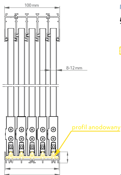
PRZEKRÓJ PIONOWY
