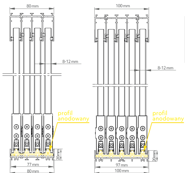
RZUT Z GÓRY SYSTEM Z USZCZELKĄ MIĘDZYSZYBOWĄ
