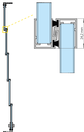
RZUT Z GÓRY SYSTEM Z LISTWAMI MIĘDZYSZYBOWYCH
