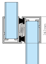
RZUT Z GÓRY SYSTEM Z USZCZELKĄ MIĘDZYSZYBOWĄ
