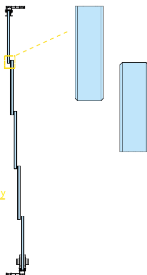
RZUT Z GÓRY SYSTEM BEZ LISTEW MIĘDZYSZYBOWYCH
